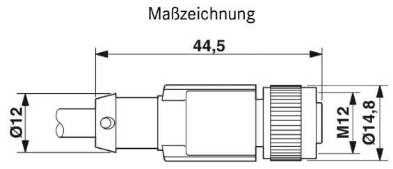
Buchse M12 x 1, gerade, geschirmt
