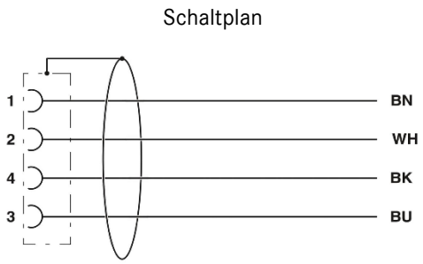
Kontaktbelegung der M12-Buchse
