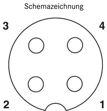
Polbild M12-Buchse, 4-polig, A-kodiert, Ansicht Stiftseite
