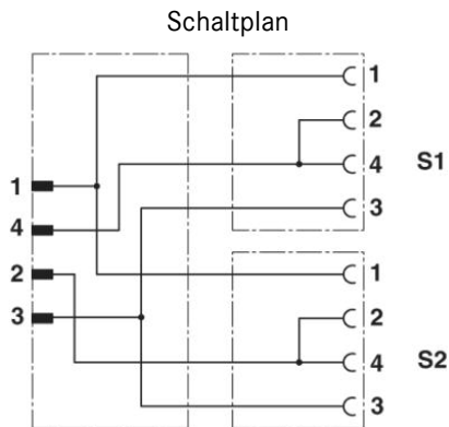
Kontaktbelegung des M12-Stecker Y und der M12-Buchse
