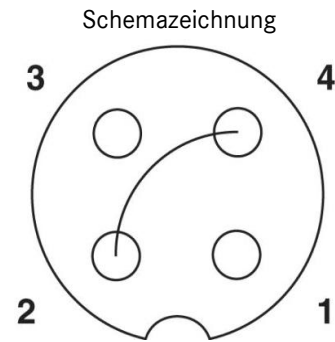
Polbild Buchse M12, 3-polig, PIN 2+4 gebrückt, A-kodiert, Ansicht Buchsenseite
