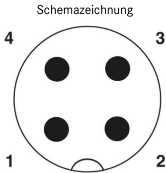
Polbild M12-Stecker Y, 4-polig, A-kodiert, Ansicht Stiftseite
