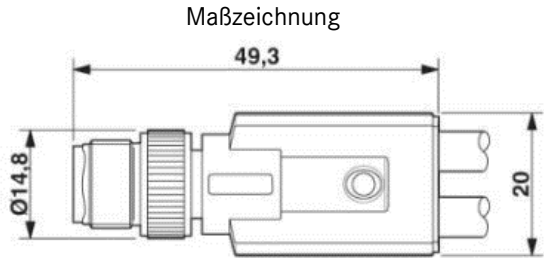
Stecker M12 x 1, Y-Verteiler
