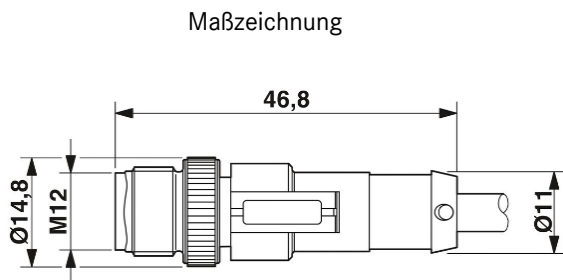
Stecker M12 x 1, gerade, A-kodiert
