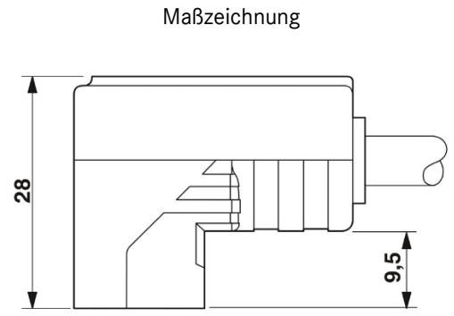
Ventilstecker, Bauform C, Seitenansicht
