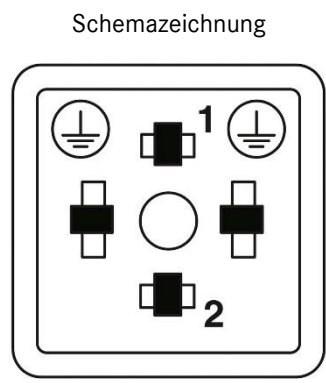
Polbild Ventilstecker, Bauform C
