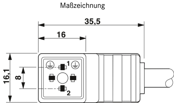
Ventilstecker, Bauform C
