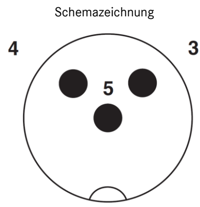
Polbild M12-Stecker, 3-polig, A-kodiert
